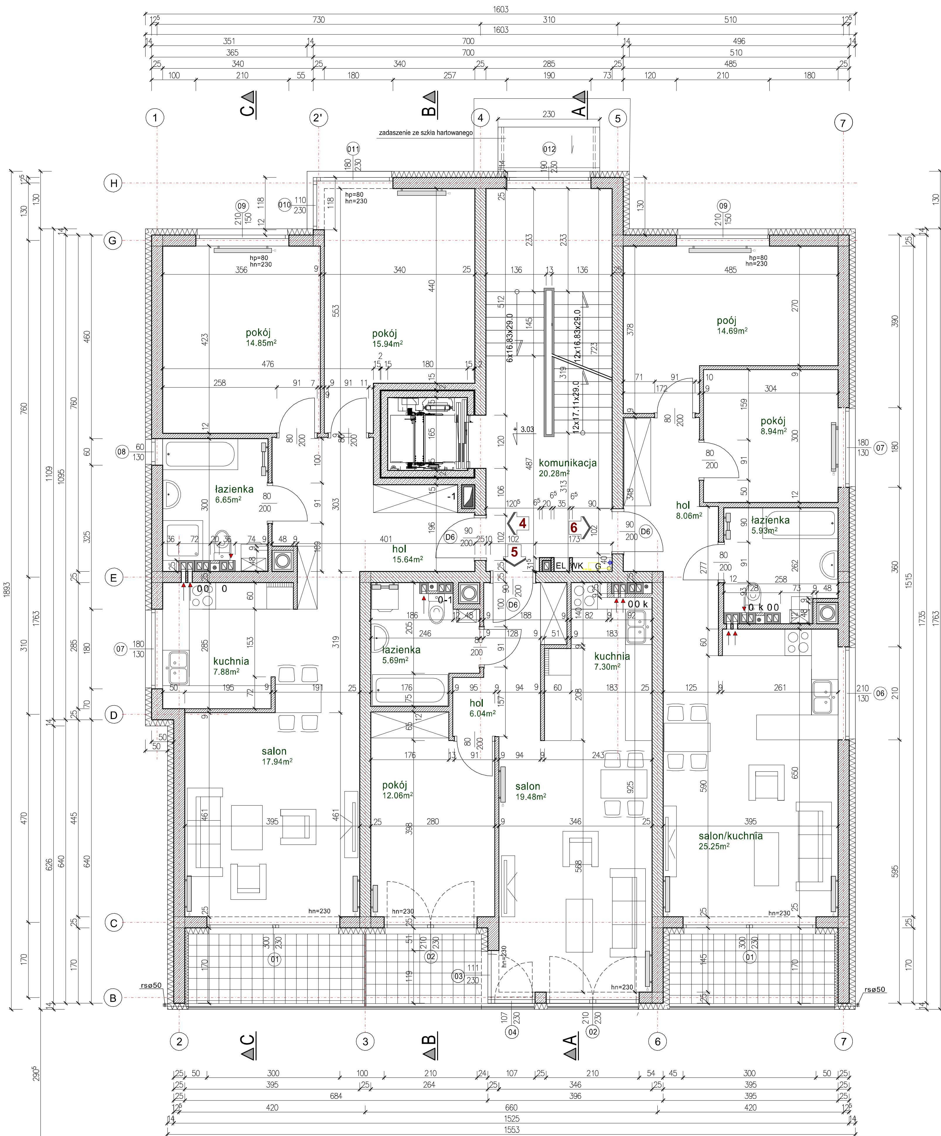
M4 MIESZKANIE NR 4 PU= 78.90 m 2
